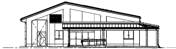
西側立面図
