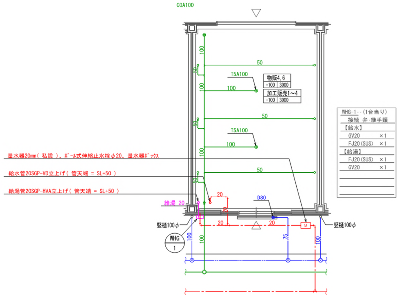
給排水設備 配管凡例
