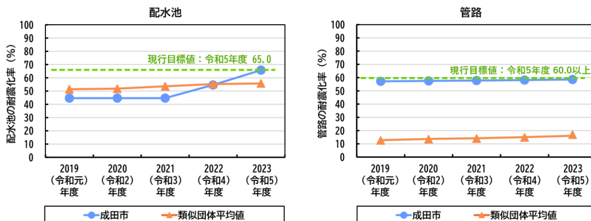
図 3.1.4 耐震化率の推移と類似団体比較
