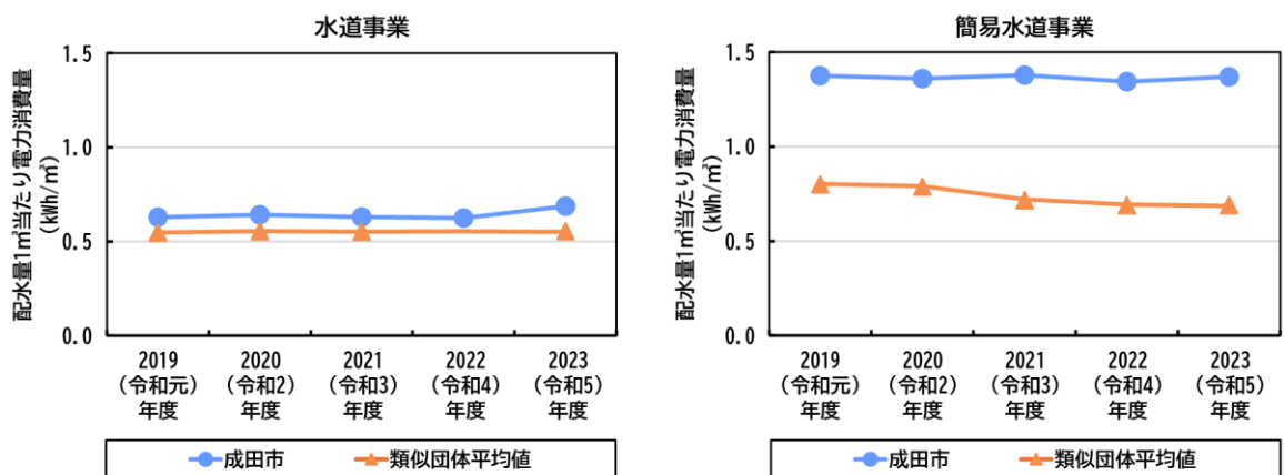
図 3.1.9 電力消費量の推移と類似団体比較
