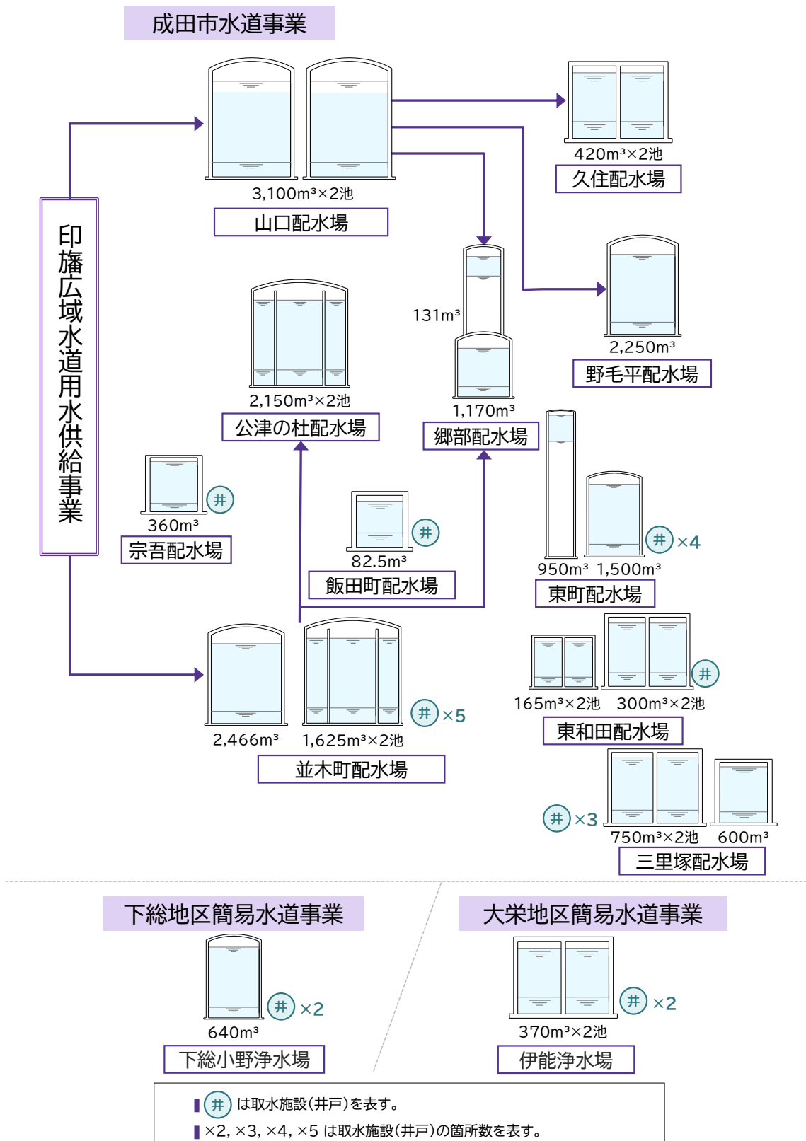
図 2.4.1 市営水道配水系統図
