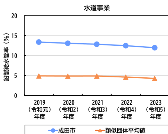
図 3.1.13 鉛製給水管率 ※ の推移と類似団体 1 比較（水道事業）
