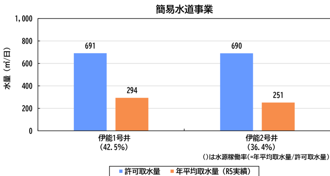
図 3.1.11 取水量が減少傾向の井戸の水源稼働率（簡易水道事業）
