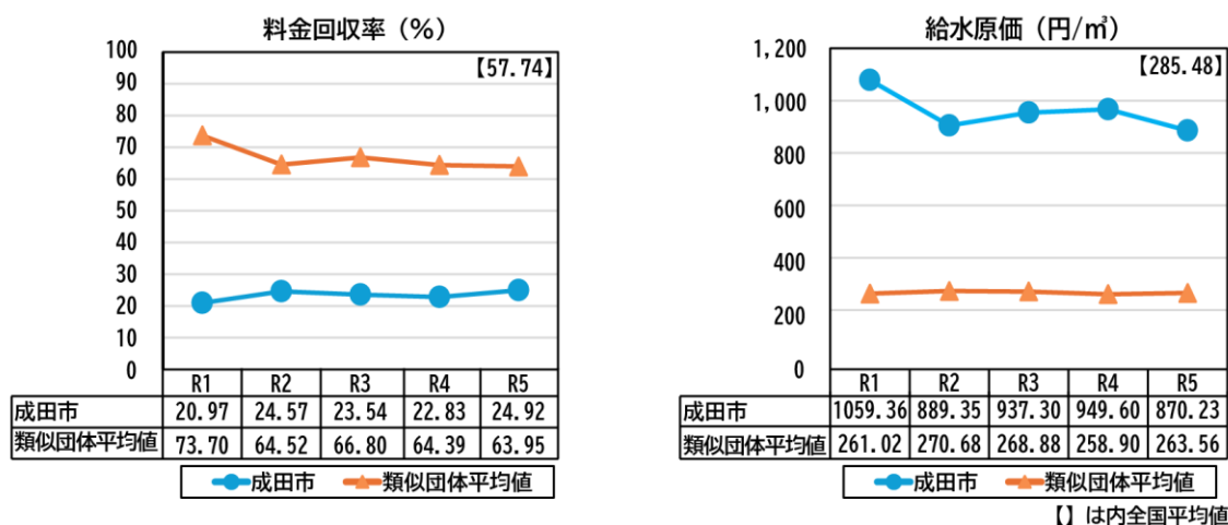
図 7.1.9 料金回収率・給水原価の推移
