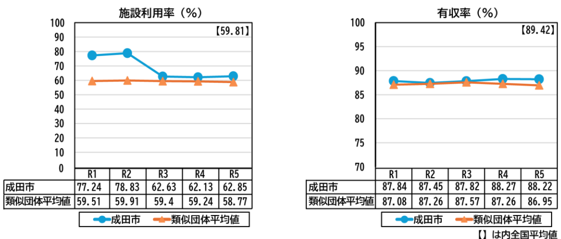
図 7.1.3 施設利用率、有収率の推移
