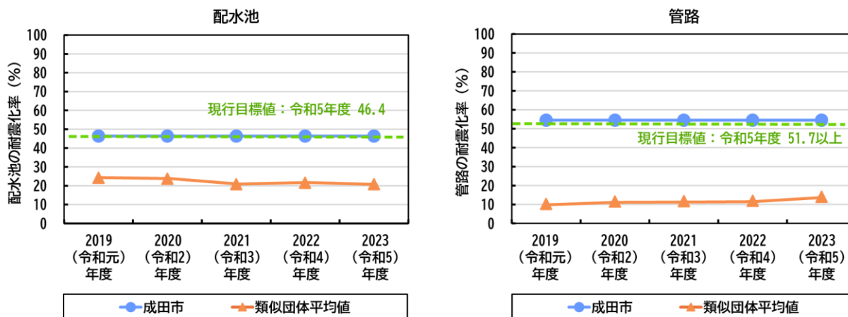
図 3.1.5 耐震化率の推移と類似団体比較
