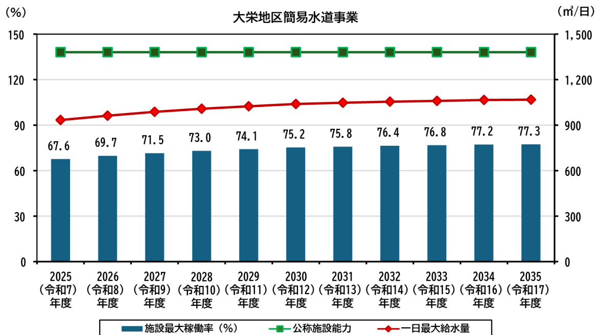
図 4.1.6 施設効率性の見通し（大栄地区簡易水道事業）
