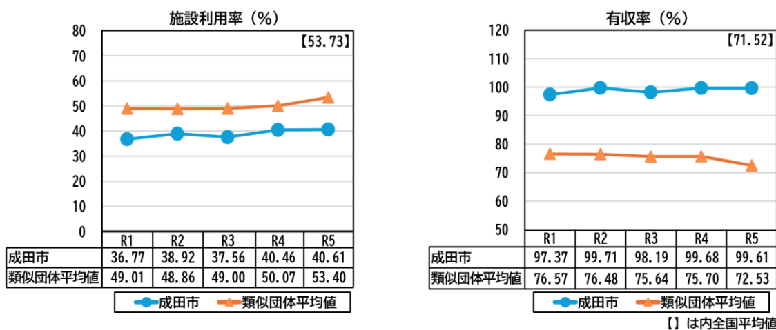
図 7.1.10 施設利用率、有収率の推移
