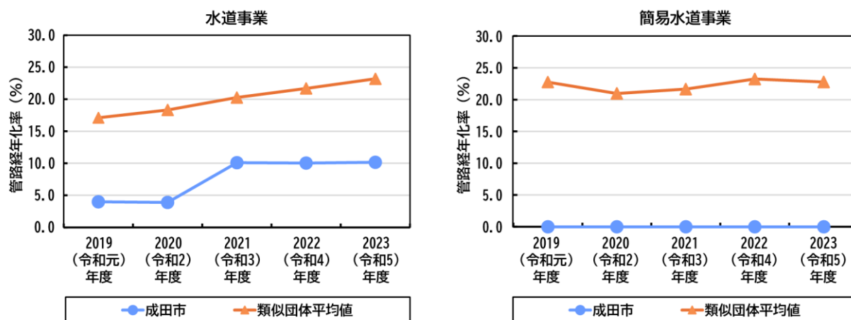
図 3.1.3 管路経年化率の推移と類似団体比較
