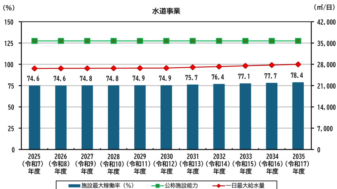
図 4.1.4 施設効率性の見通し (水道事業)
