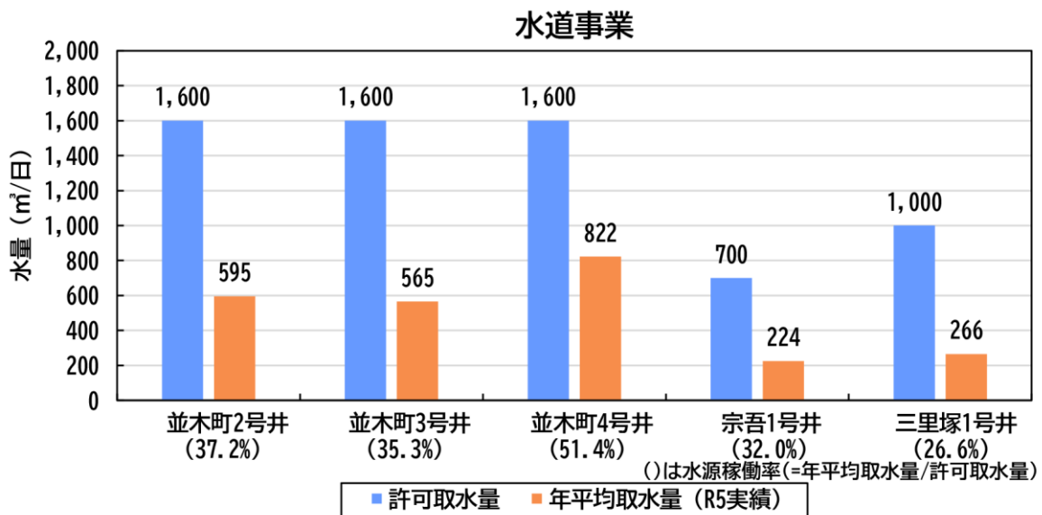
図 3.1.10 取水量が減少傾向の井戸の水源稼働率（水道事業）
