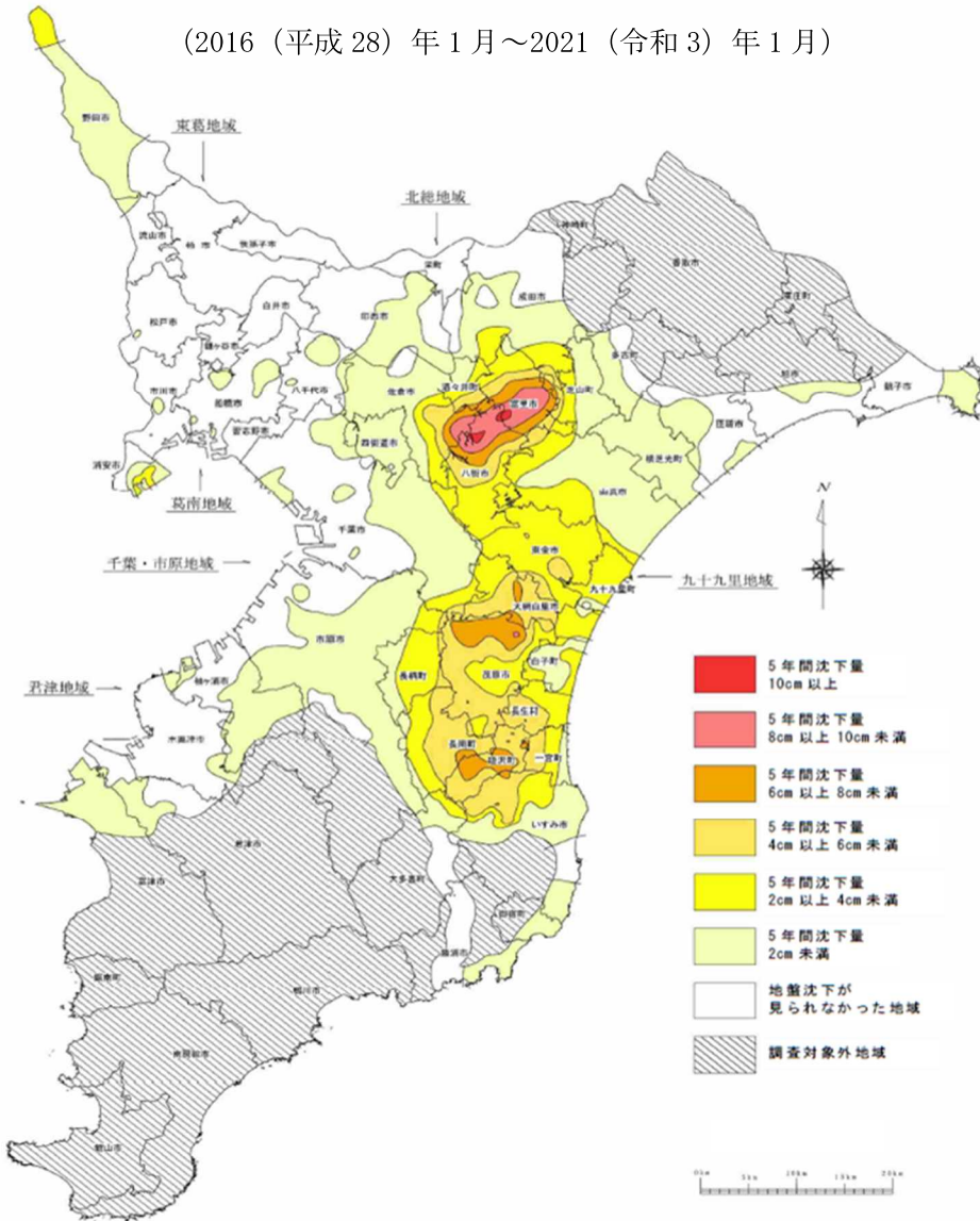
図 2-5-1 千葉県水準基標変動図 (5 年間変動図)
