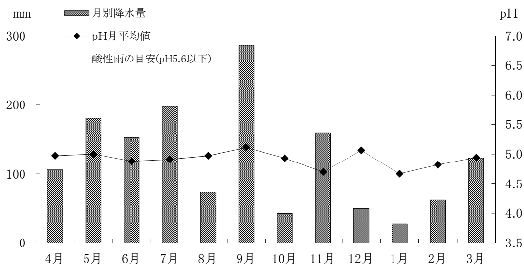
図 4-13 2018 (平成 30) 年度の月別降水量と酸性度
