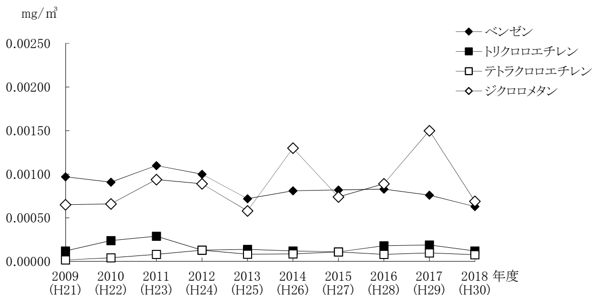
図 4-12 有害大気汚染物質濃度の年平均値の推移
