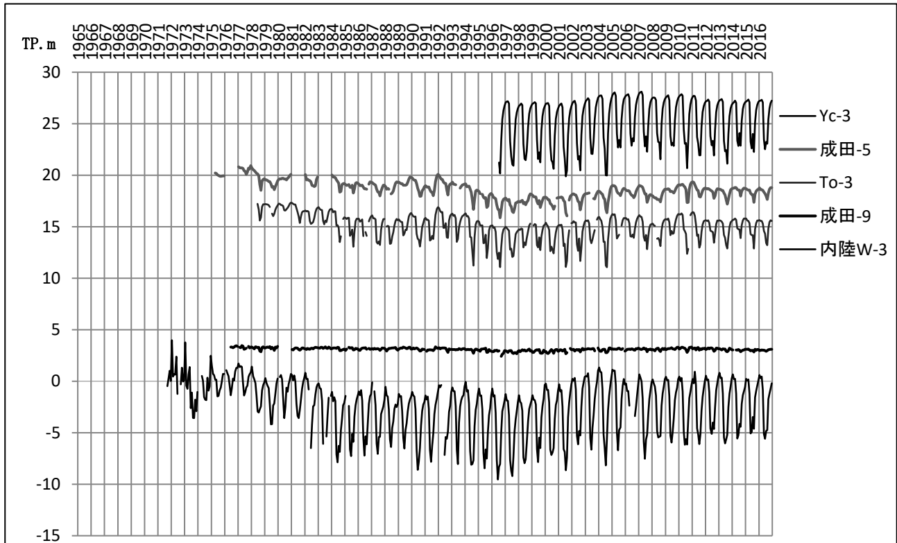
図 8-5 主要地点の地下水位変動図
