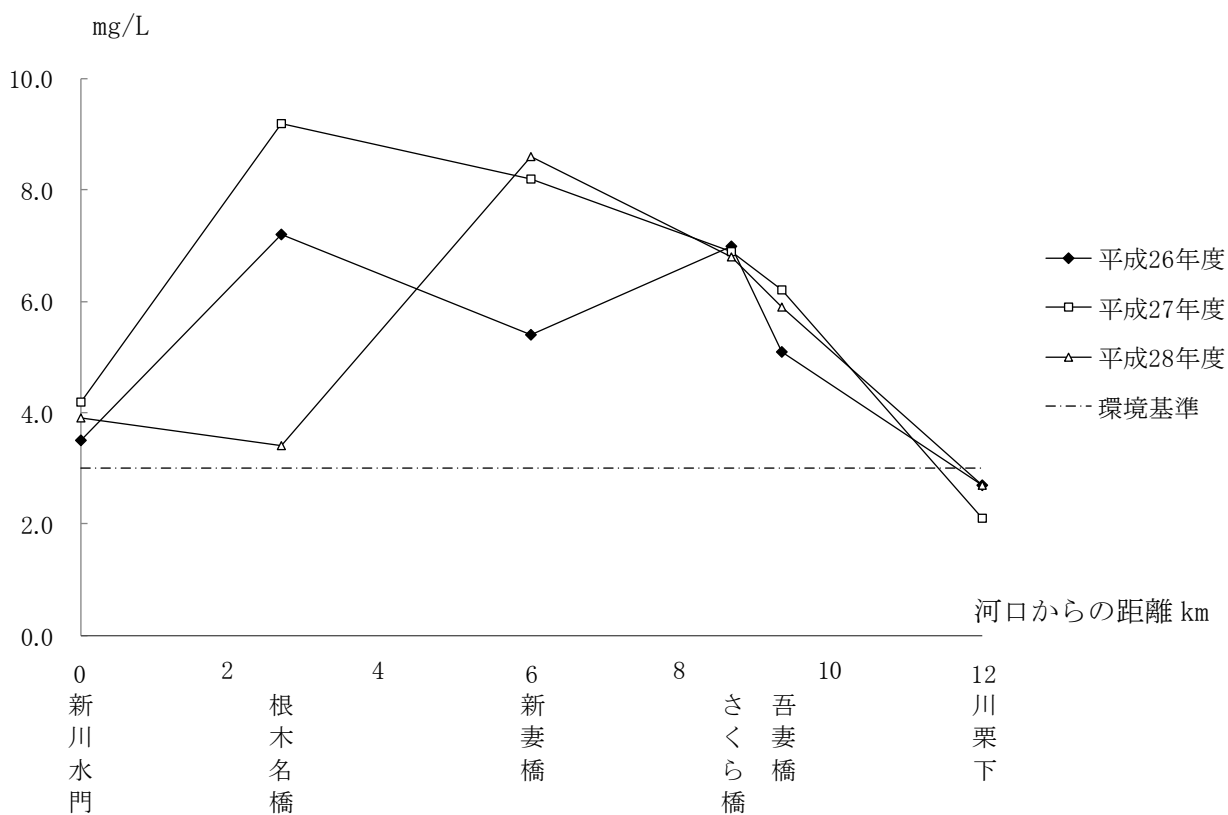
図 5-3 根木名川 BOD (75%値) 縦断変化
