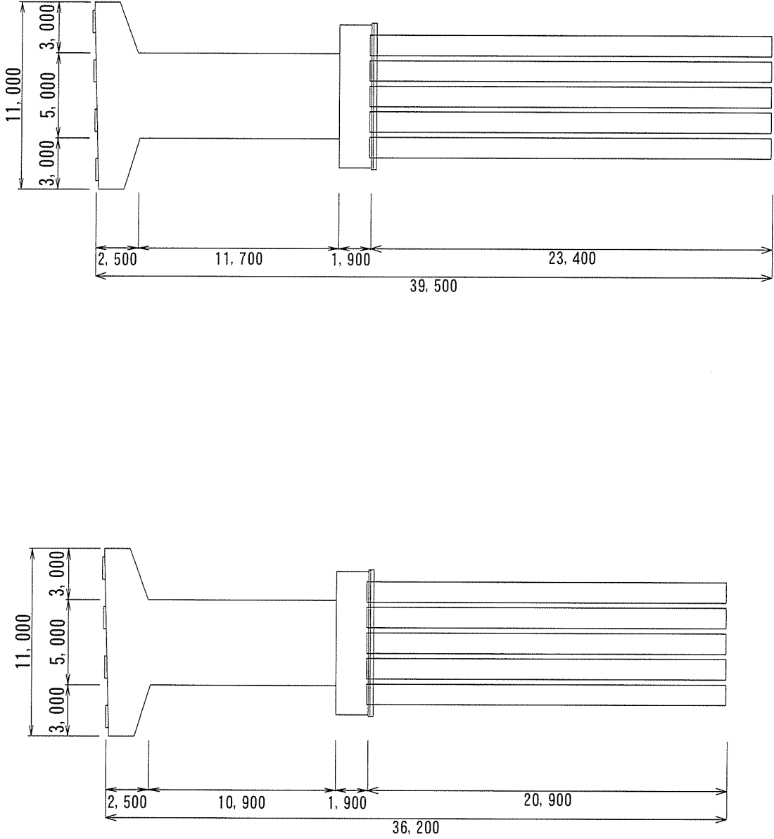
橋脚 A
