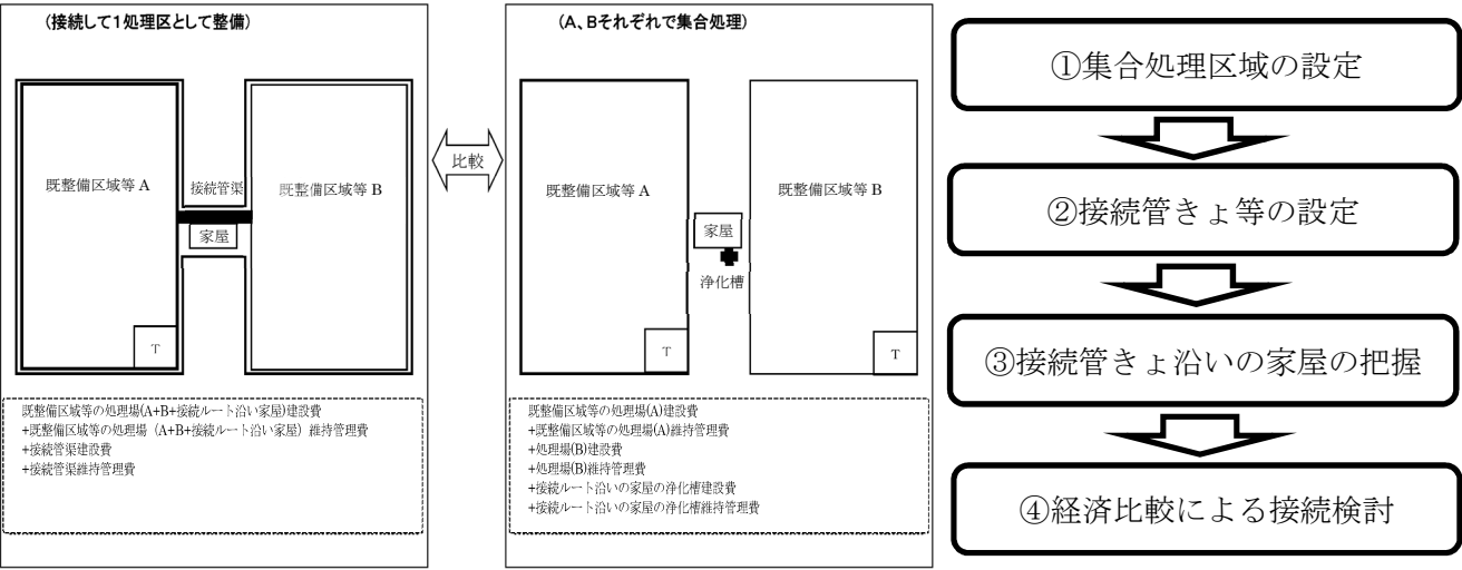
図-4 集合処理区域同士の接続検討の概念図 出典：千葉県マニュアル
