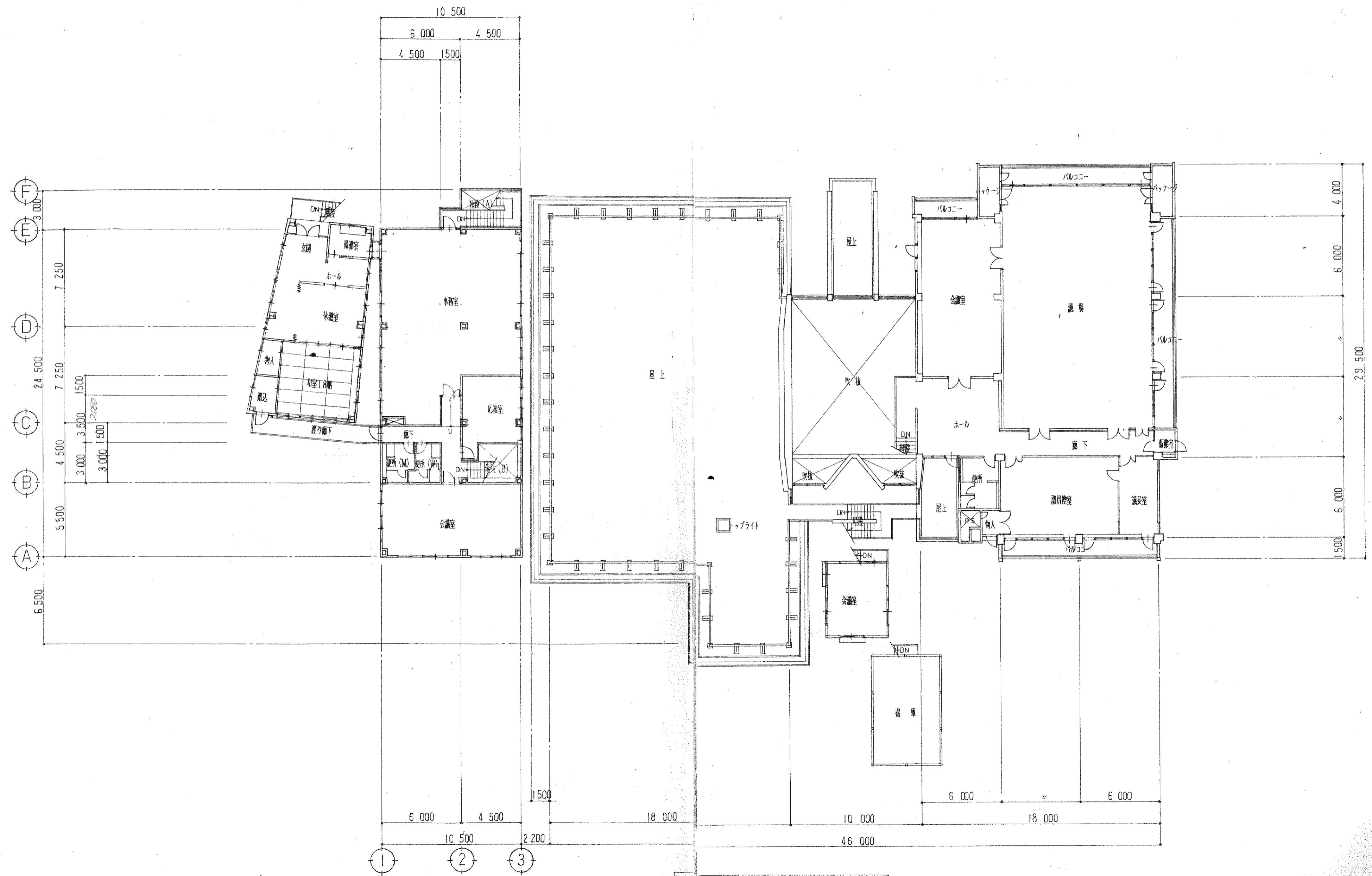
2階平面図 1:200
