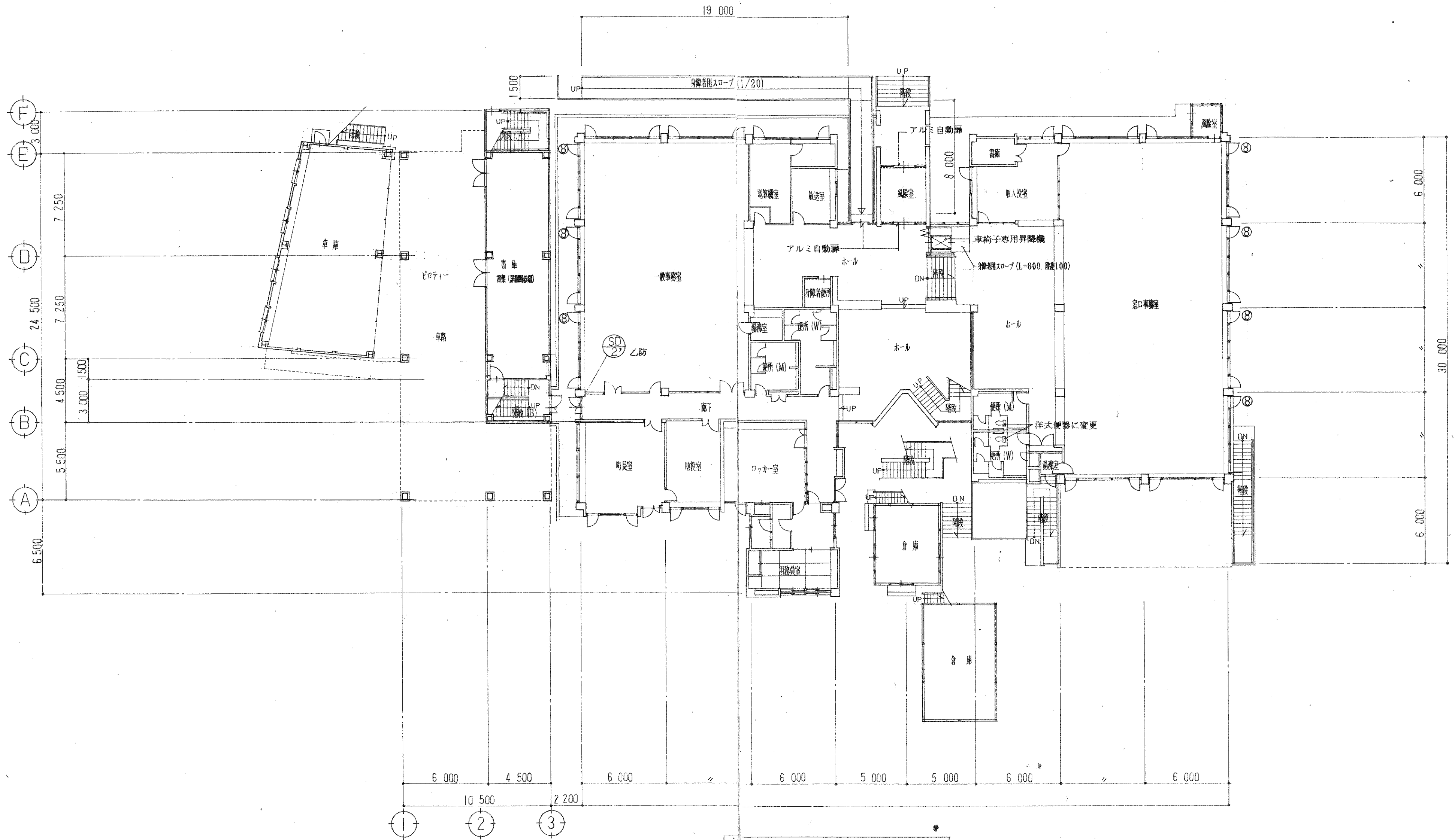
1階平面図 1:200
