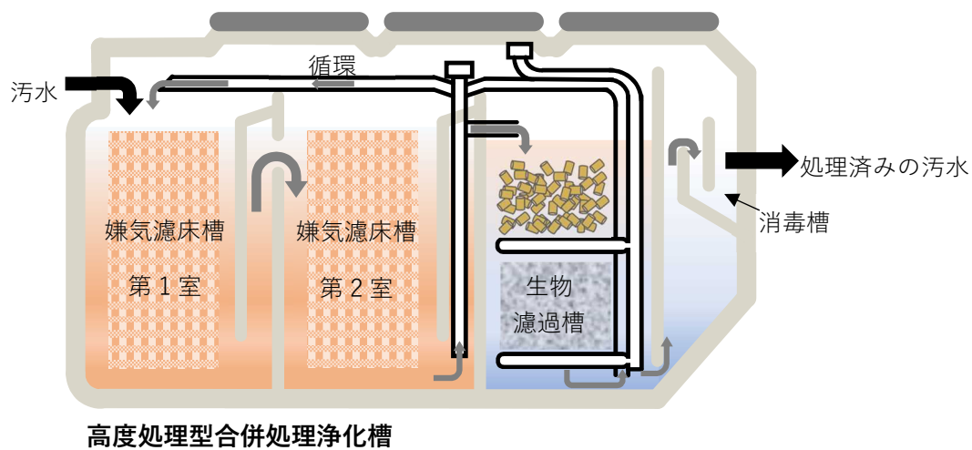
【図 23】 合併処理浄化槽の構造（模式図）
