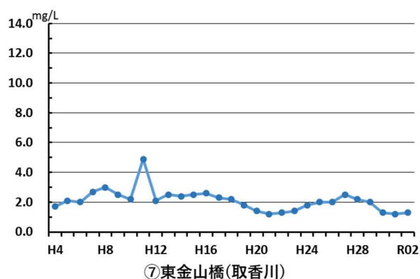
【図 10】 根本名川に流入する河川の各測定地点の測定値（BOD 75%値）
