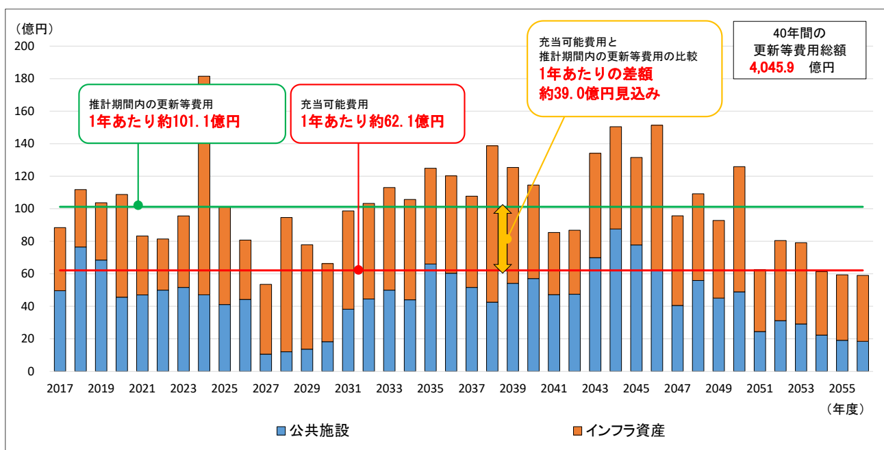
図 2-20 公共施設等の将来の更新等費用推計グラフ（特別会計含む）
