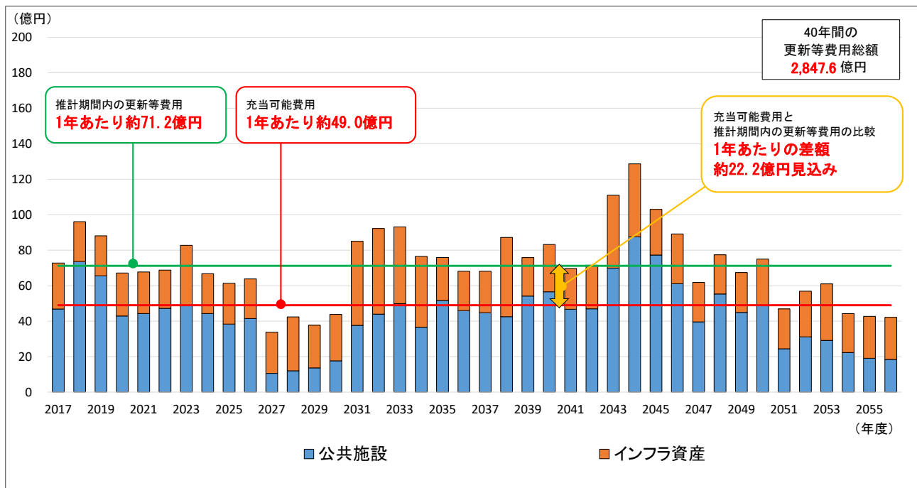
図 2-19 公共施設等の将来の更新等費用推計グラフ（一般会計のみ）
