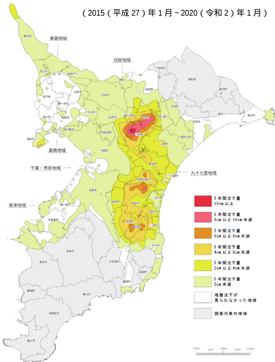
図2-5-1 千葉県水準基標変動図(5年間変動図)
