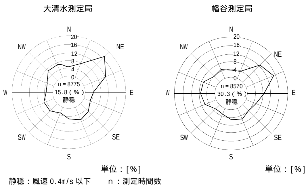
図 2 - 1 - 4 風配図
