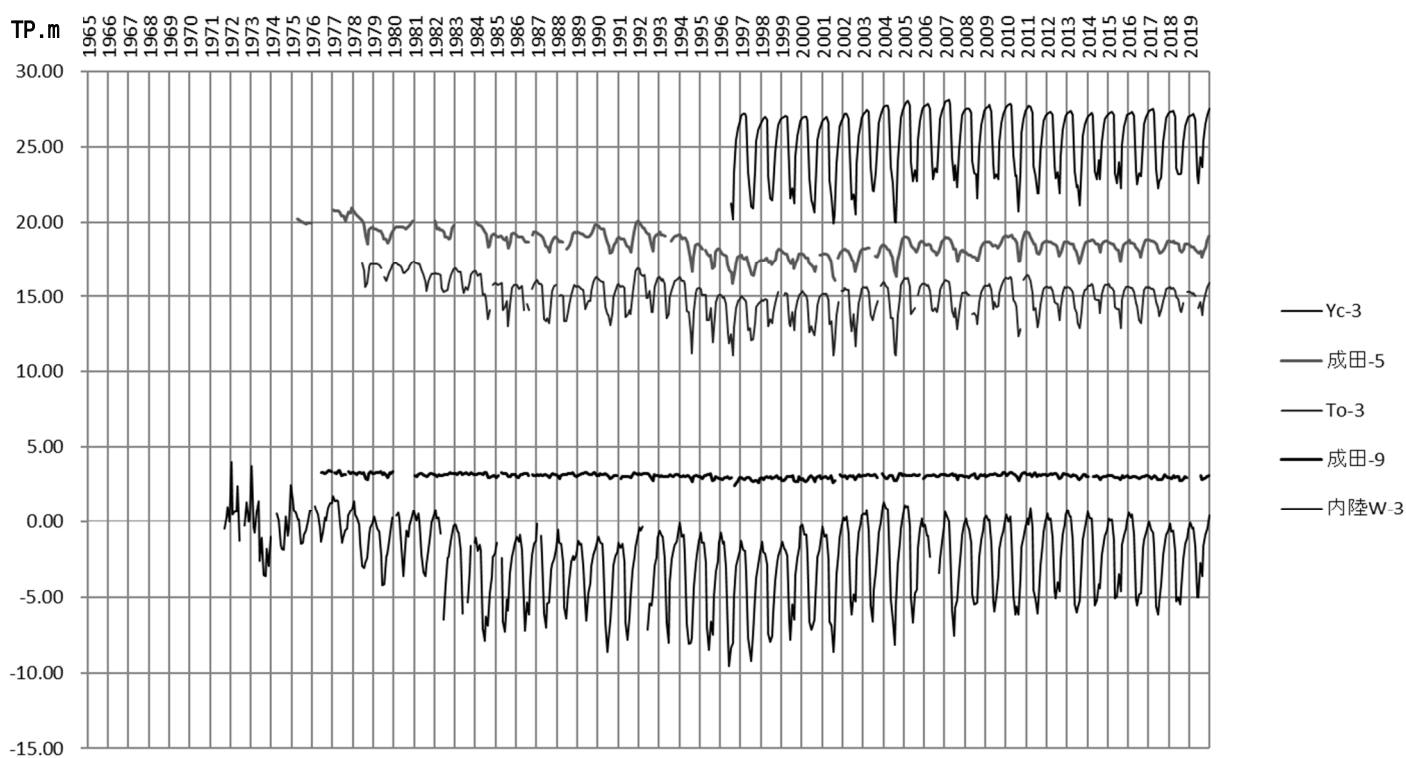
図 2 - 5 - 5 主要地点の地下水位変動図
