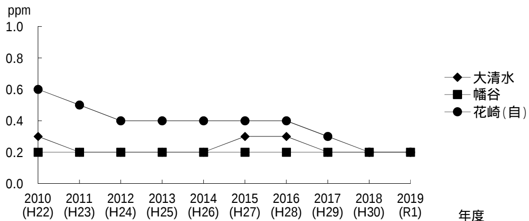
図 2 - 1 - 10 一酸化炭素濃度の年平均値の推移
