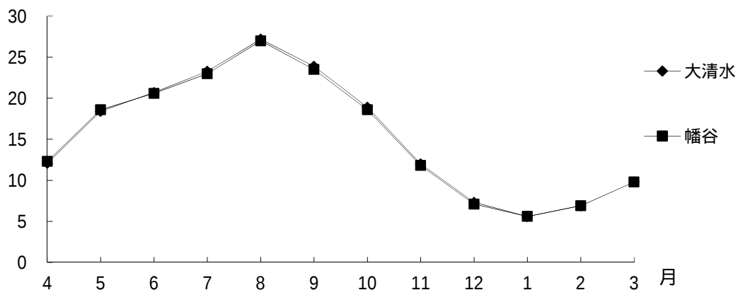
図 2 - 1 - 2 気温の月平均値の推移（大清水、幡谷測定局）
