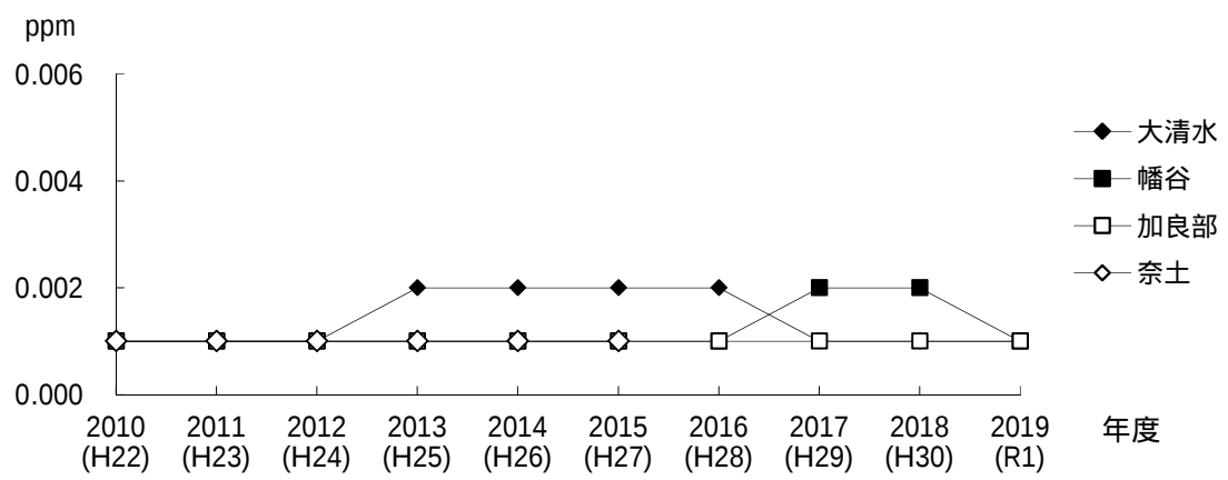
図 2 - 1 - 5 二酸化硫黄濃度の年平均値の推移
