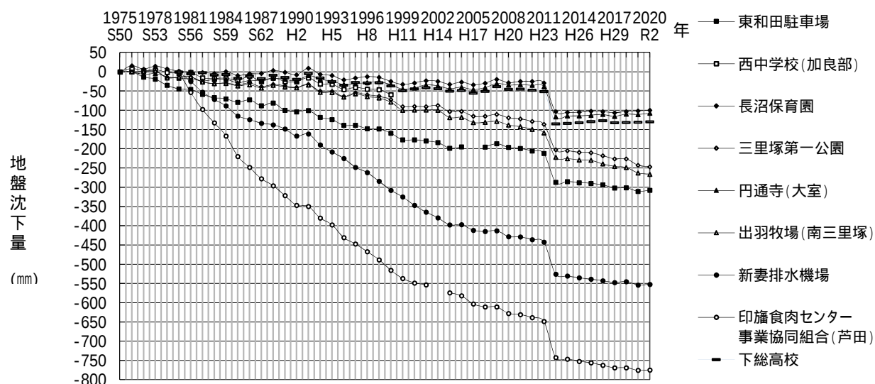
図 2 - 5 - 4 市内主要水準点の経年地盤変動傾向図
