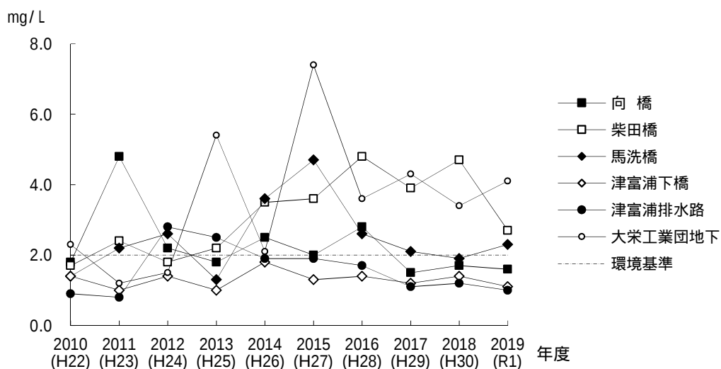
図 2 - 2 - 11 根木名川 B O D 年平均値の推移
