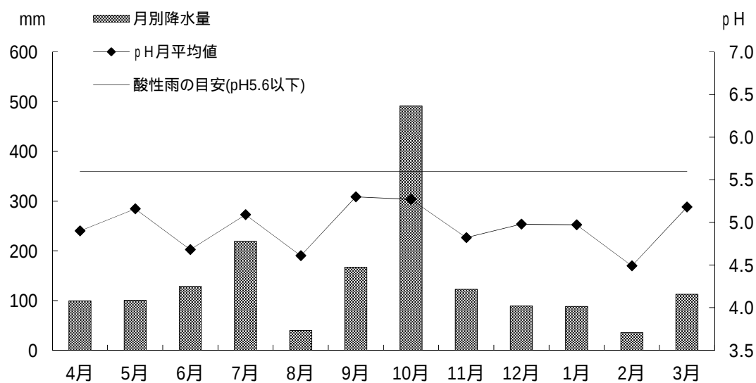
図 2 - 1 - 13 2019 ( 令和元 ) 年度の月別降水量と酸性度
