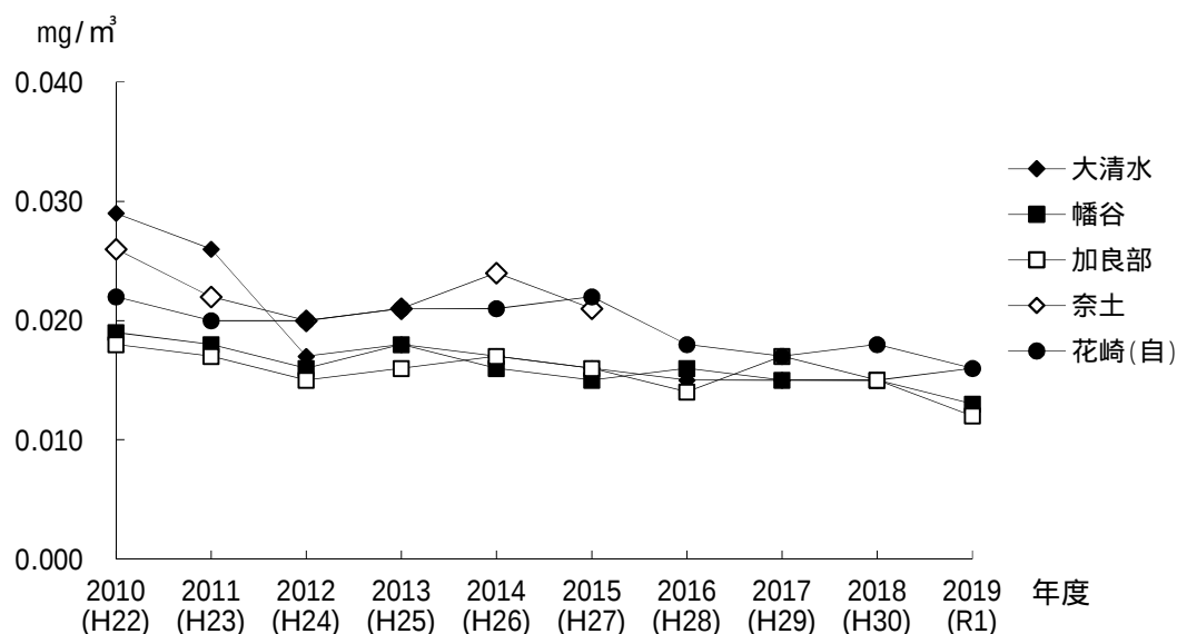
図 2 - 1 - 11 浮遊粒子状物質濃度の年平均値の推移
