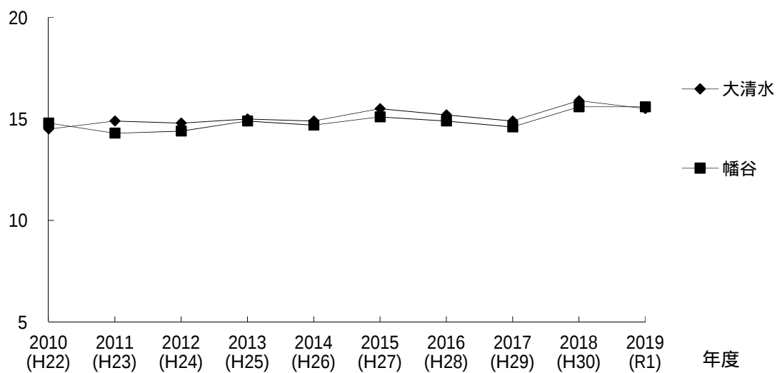
図 2 - 1 - 3 気温の年平均値の推移（大清水、幡谷測定局）
