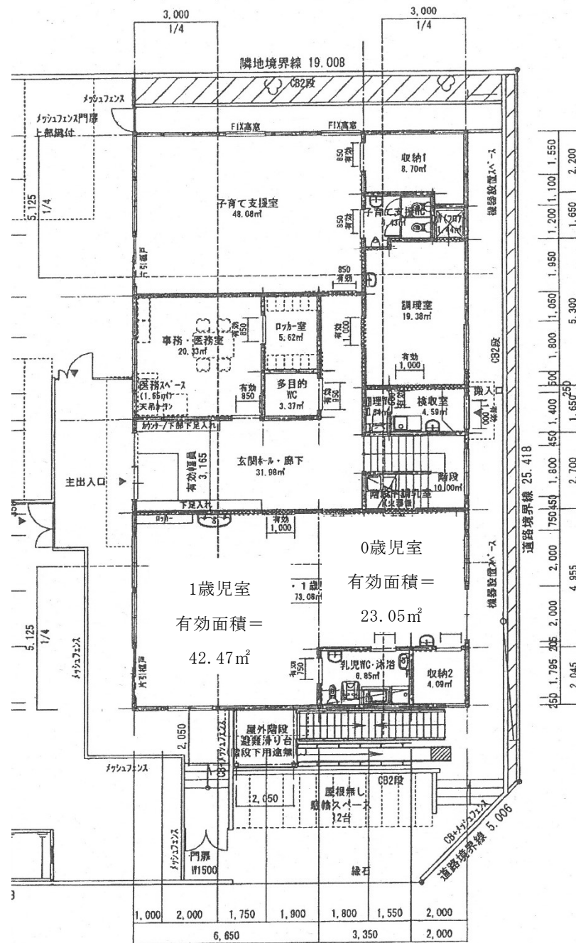
1 階平面図
