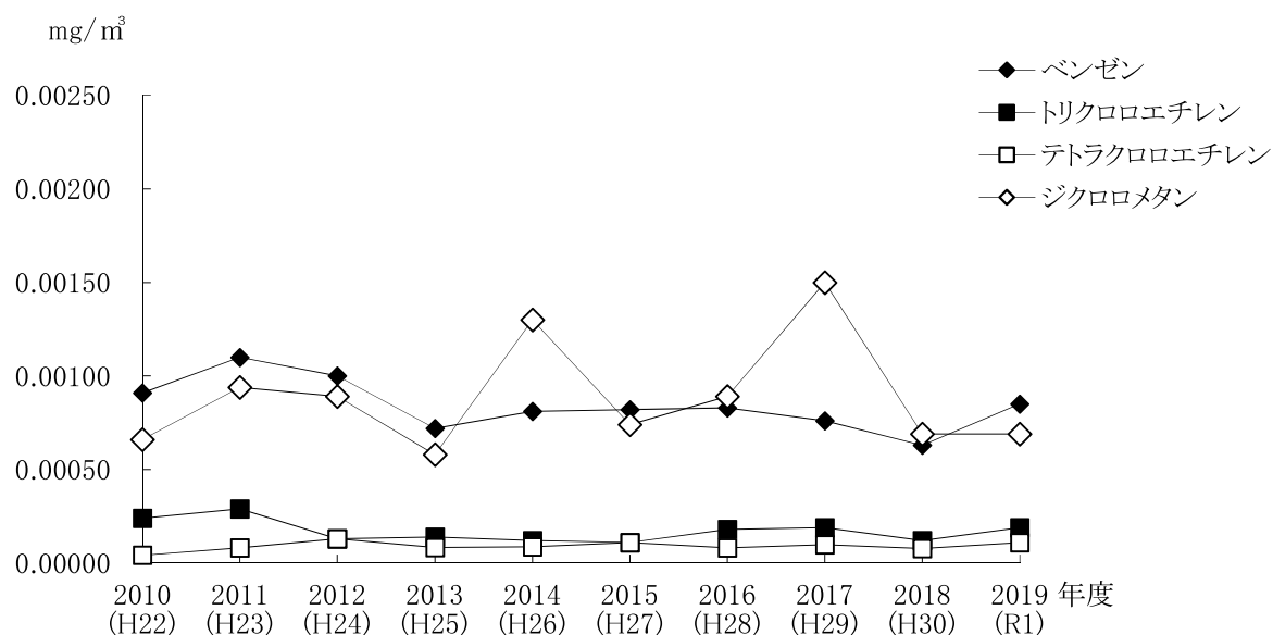
図 2-1-12 有害大気汚染物質濃の年平均値の推移
