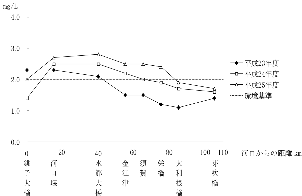
図 5-2 利根川 BOD（75%値） 縦断変化
