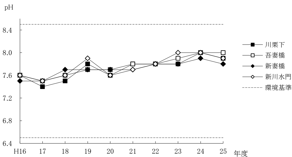
図 5-4 根木名川 pH 年平均值の推移
