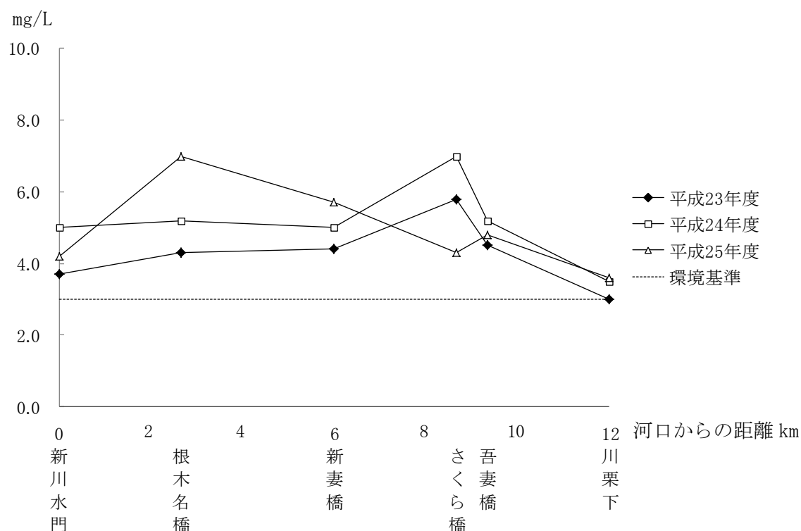
図 5-3 根木名川 BOD (75%値) 縦断変化
