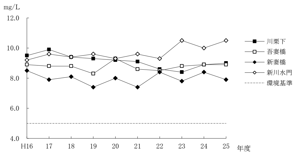
図 5-7 根木名川DO 年平均値の推移
