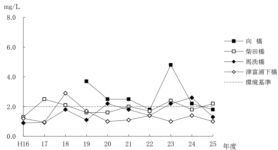
図 5-10 根木名川 BOD 年平均値の推移
