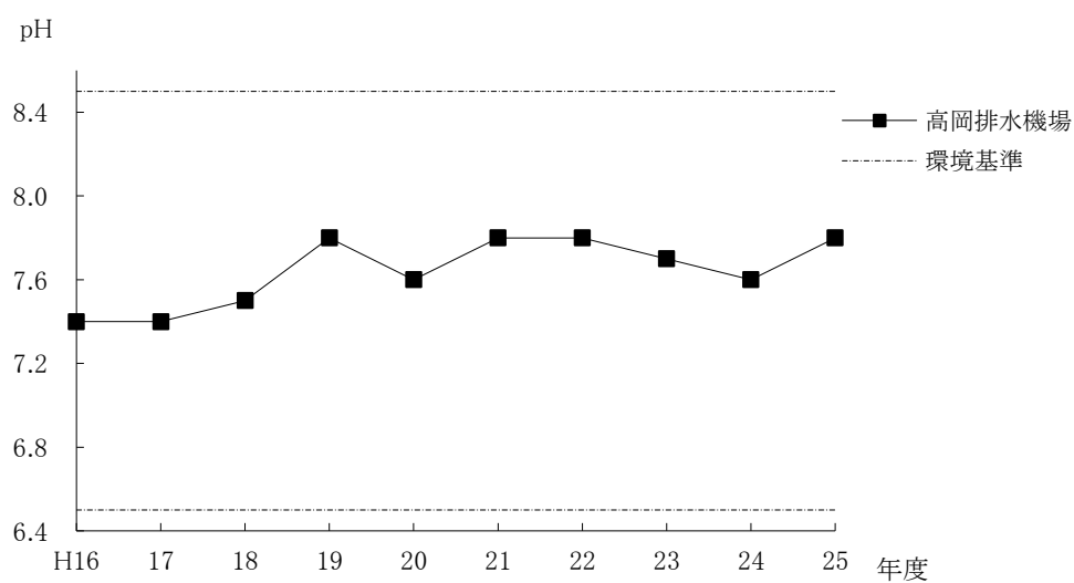
図 5-5 大須賀川 pH 年平均值の推移
