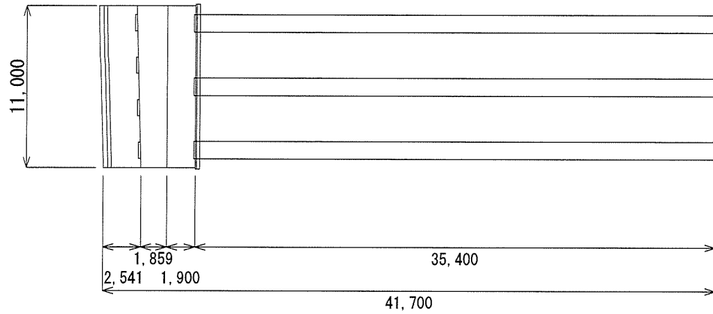
橋台B
