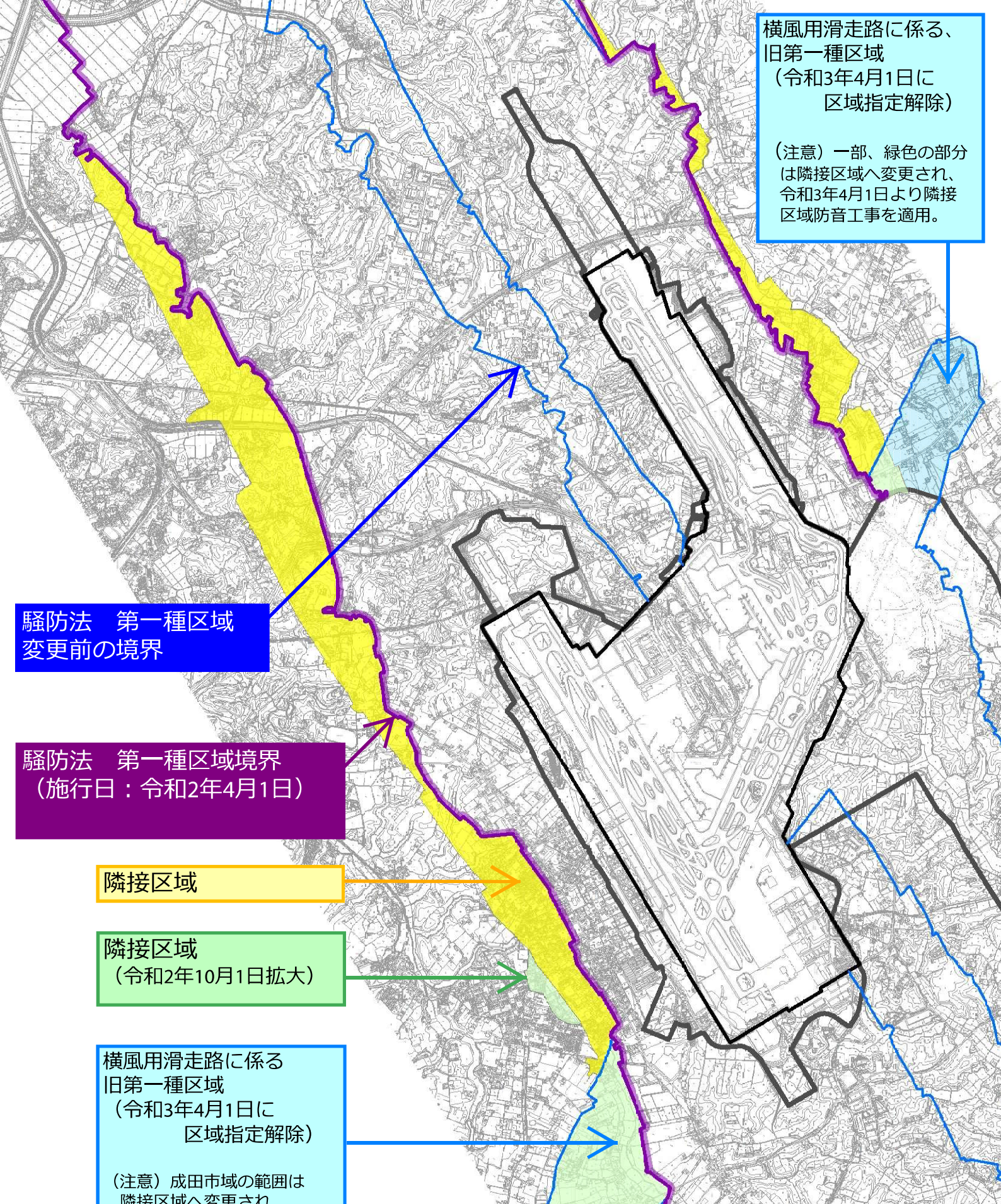
第一種区域・ 隣接区域図 (成田市南側)
