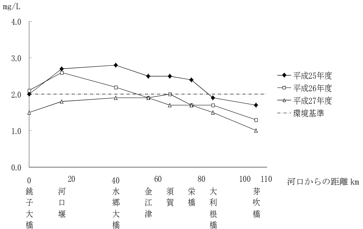
図 5-2 利根川 BOD (75% 値) 縦断変化
