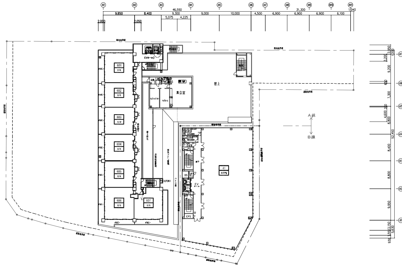
施設・住宅棟 6階平面図
