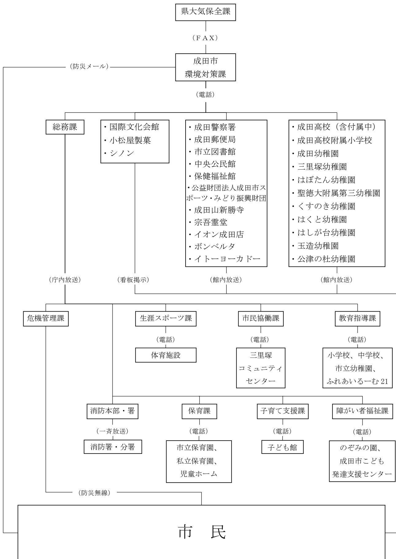
図 4-9 成田市光化学スモッグ情報連絡体制組織図 (平日・平成 24 年度現在)
