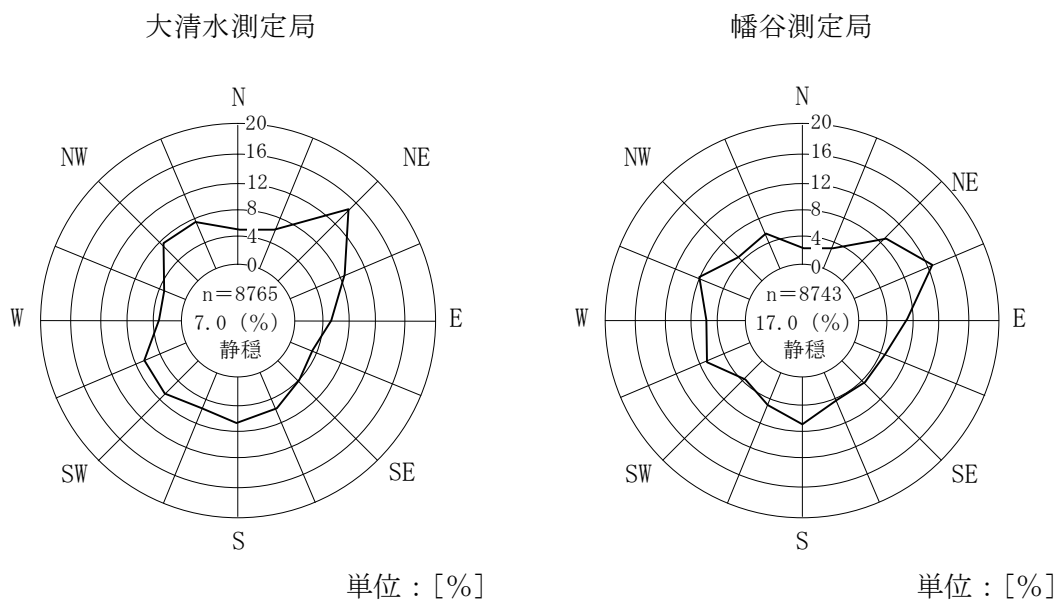
図 4-4 風配図
