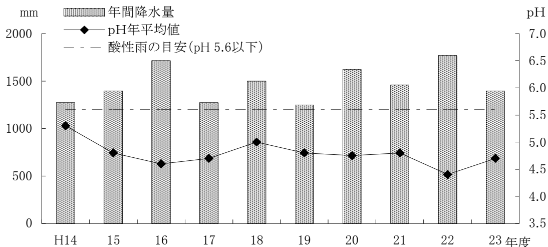
図 4-14 年間降水量と酸性度の推移
