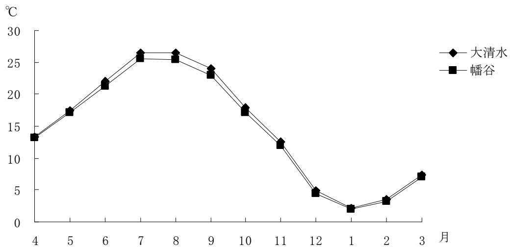
図4-2 気温の月平均値の推移（大清水、幡谷測定局）
