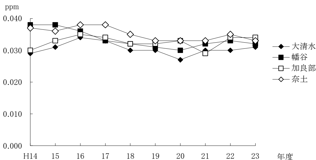
図 4-8 光化学オキシダント濃度の年平均値の推移
