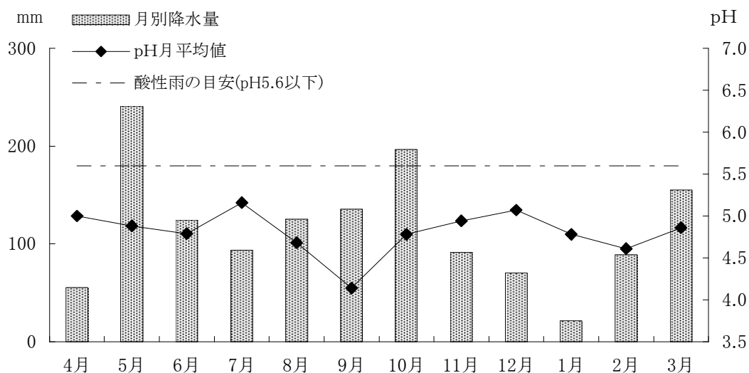
図 4-13 平成 23 年度の月別降水量と酸性度
