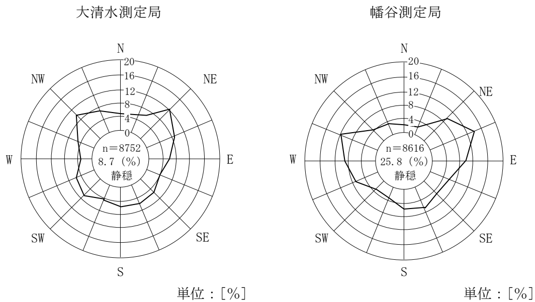
図 4-4 風配図
